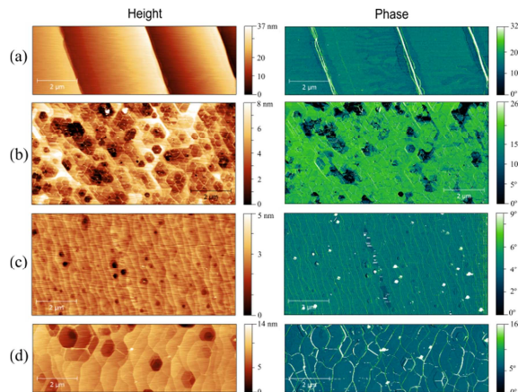
Figura 3 Imágenes AFM (altura en nm y de fase en grados). En todos los casos la escala de longitud es la misma y se utilizó un único escalón de recocido. (a) recocido a 1750 °C for 2700 s con método FTF. Las muestras mostradas en (b), (c), and (d) fueron crecidas con la cara de Si abierta, esto es, expuesta a 101 kPa de Ar usado como gas de fondo del horno. En cada caso el recocido fue (b) 1750 °C for 2700 s, (c) 1800 °C for 600 s y (d) 2000 °C por 600 s.
